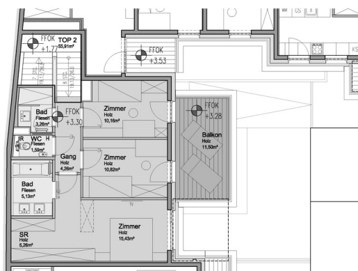
1. OBERGESCHOSS
